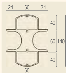
Schema tecnico
